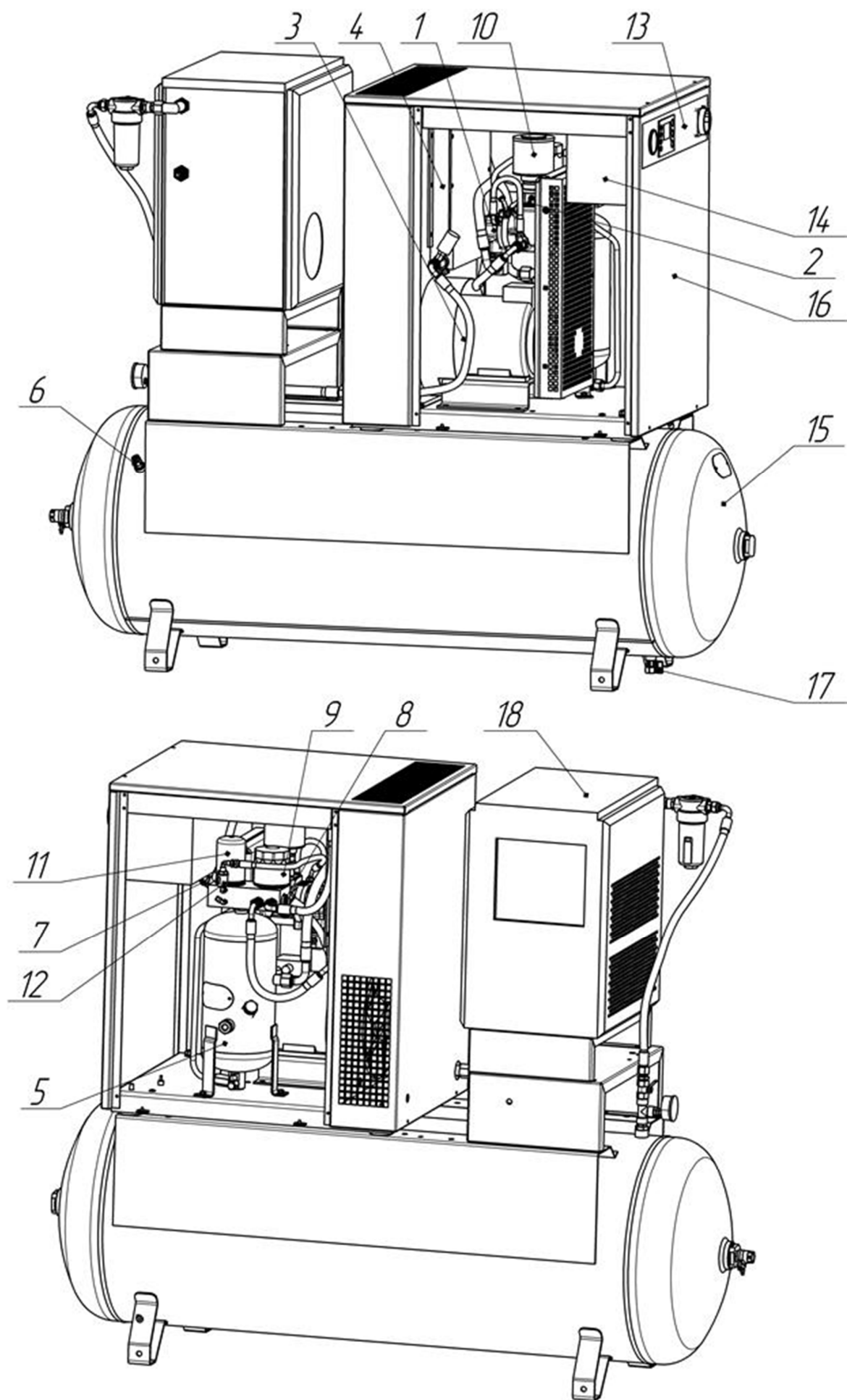
Рисунок 3 – Общий вид компрессорной установки ВК5(7, 10)Е-...-500(Д)
