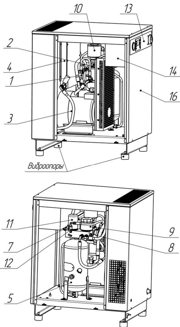
Рисунок 1 – Общий вид компрессорной установки ВК5(7, 10)Е-...
