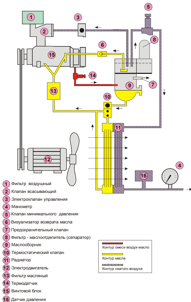
Рисунок 4 – Схема функциональная принципиальная компрессорных установок VK5 (7, 10)E
