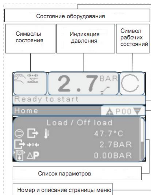
Рисунок В.1 - Дисплей контроллера
