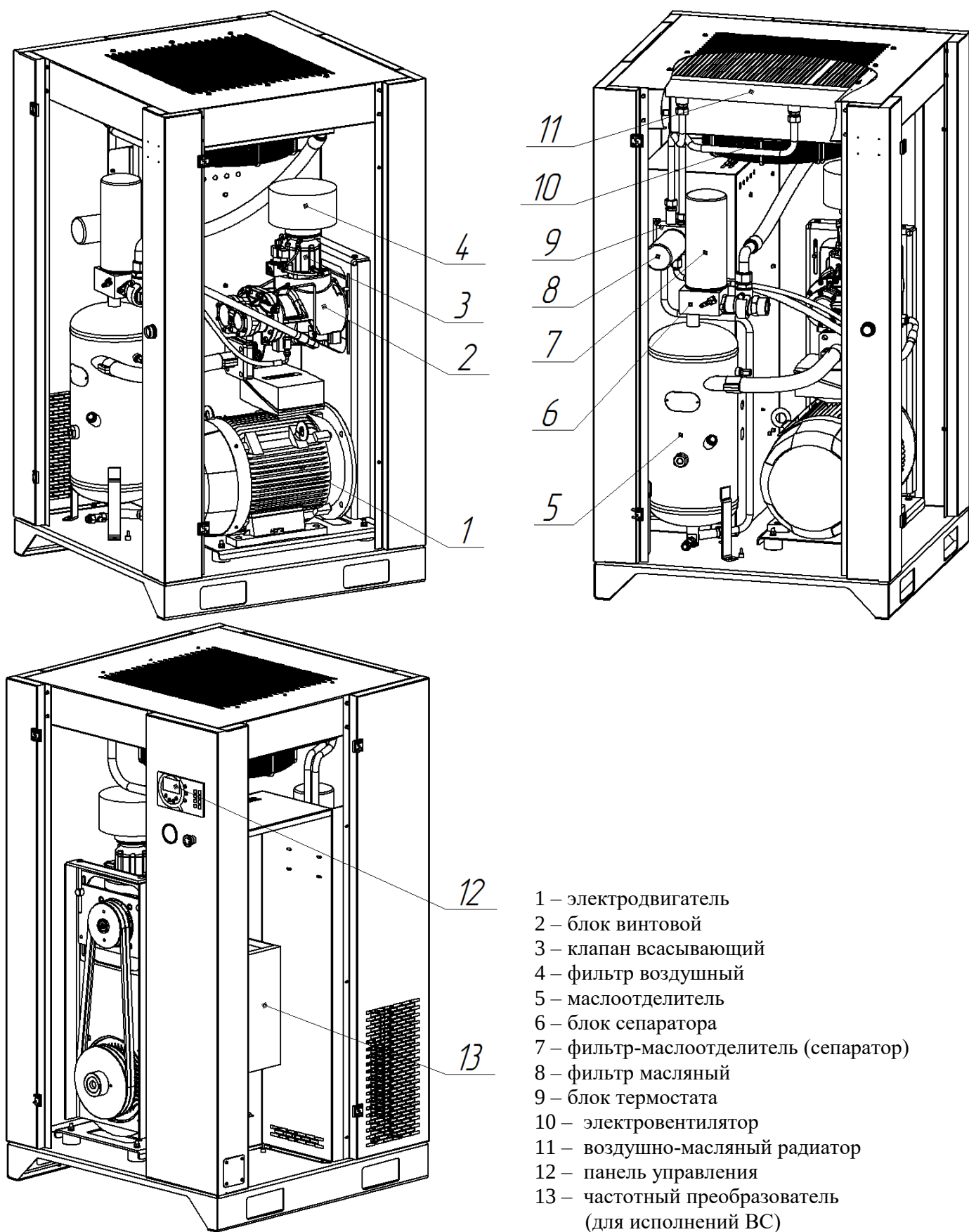
Рисунок 2 – Основные узлы установки
