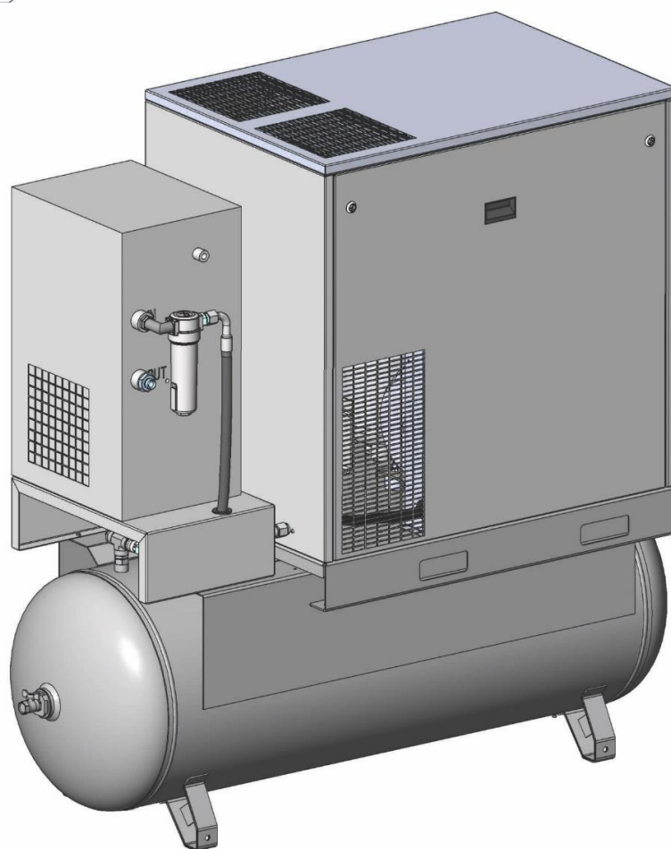
Рисунок 3 – Общий вид компрессорной установки ВК20-...-500Д(ВС)
