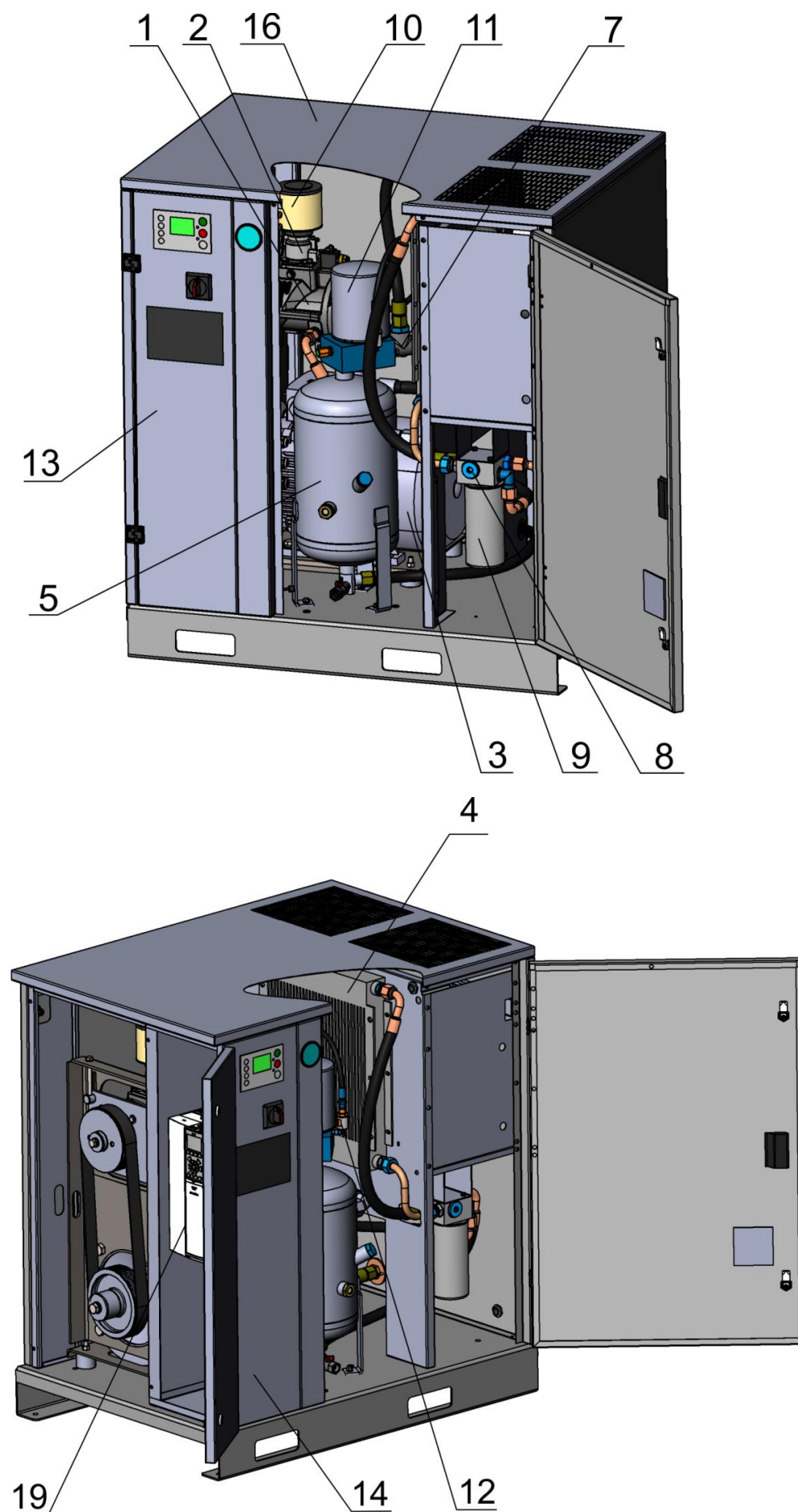
Рисунок 1 – Общий вид компрессорной установки ВК20-...(BC)
