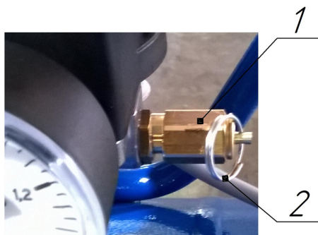
Рисунок 8 – Клапан предохранительный пружинного типа
