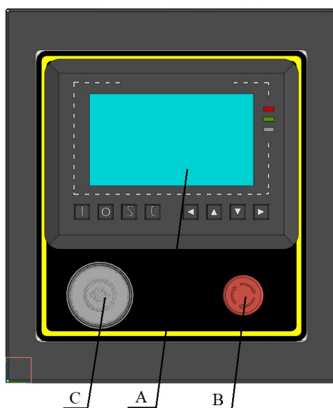
Рис. 3а – Контроллер MAM6090
