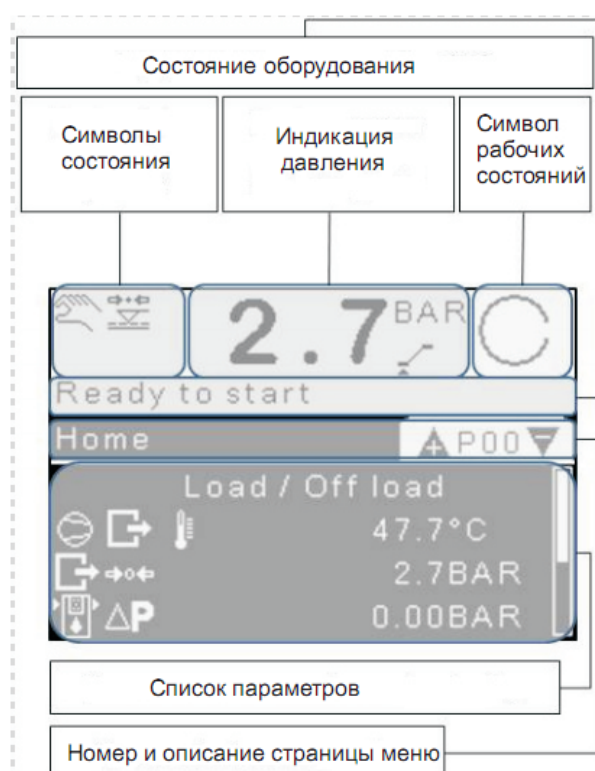
Рис. 1. Дисплей контроллера
