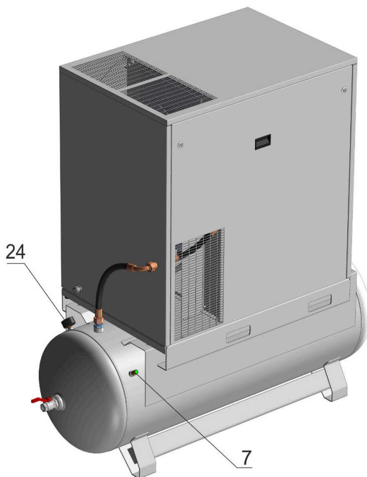
Рисунок 2 – Общий вид компрессорных установок ВК25-...-500(BC), ВК30-...-500(BC)
