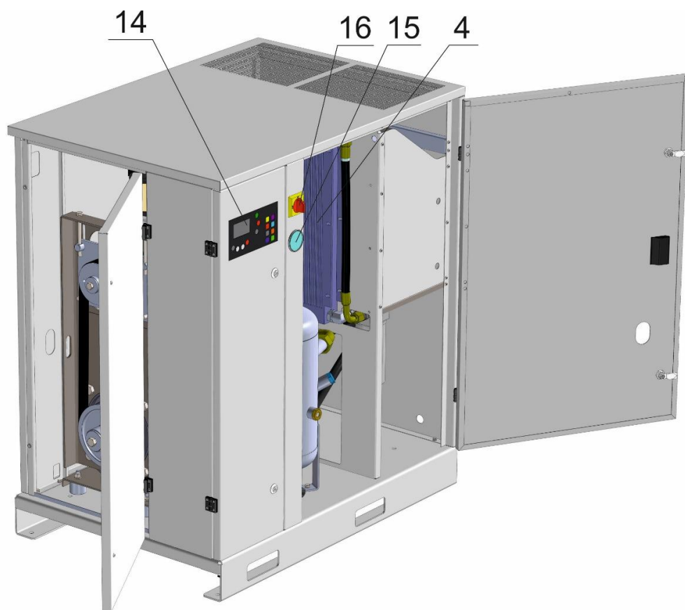
Рисунок 1 – Общий вид компрессорной установки ВК25-...(BC), ВК30-...(BC)
