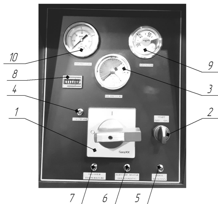
Рис. 3. Панель управления
