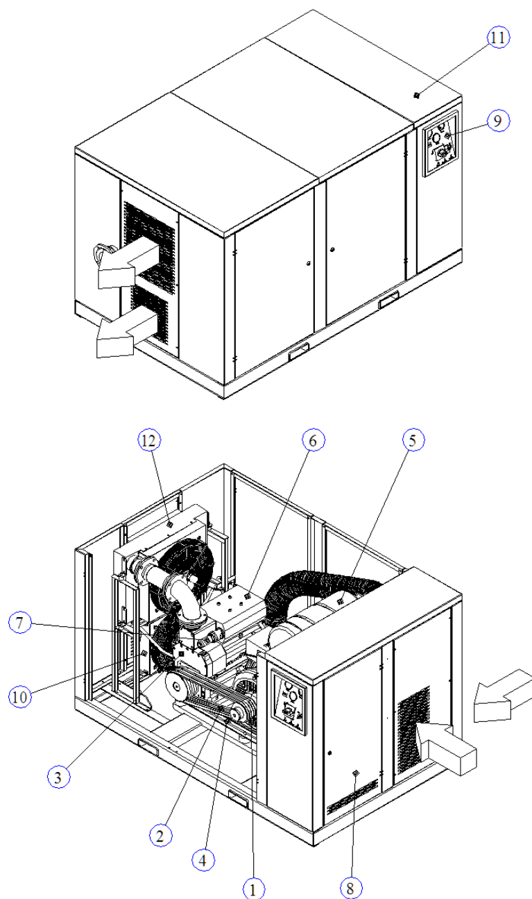
Рис. 2. Общий вид установки
