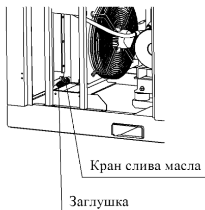
Рис. 6. Маслоохладитель
