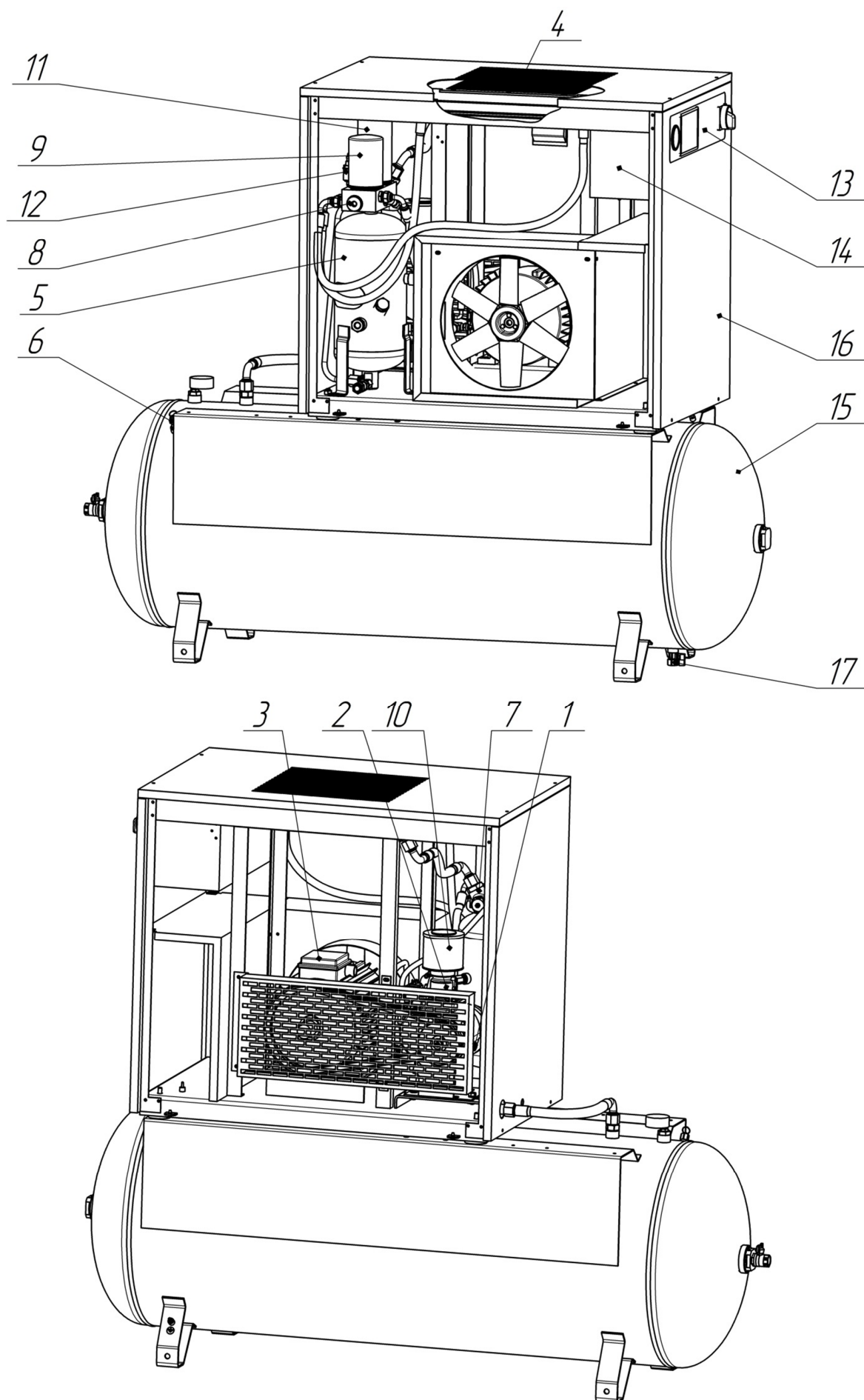
Рисунок 2 – Общий вид компрессорной установки ВК15Е-...-500
