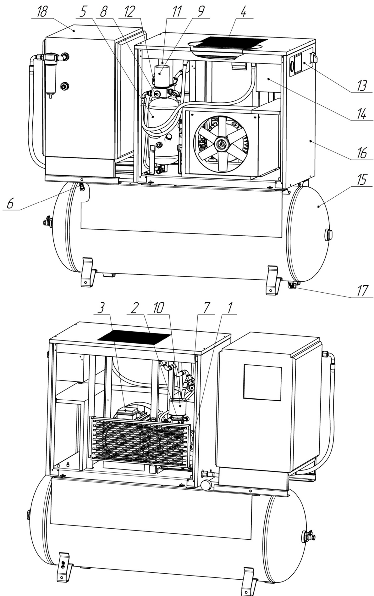
Рисунок 3 – Общий вид компрессорной установки ВК15Е-...-500Д
