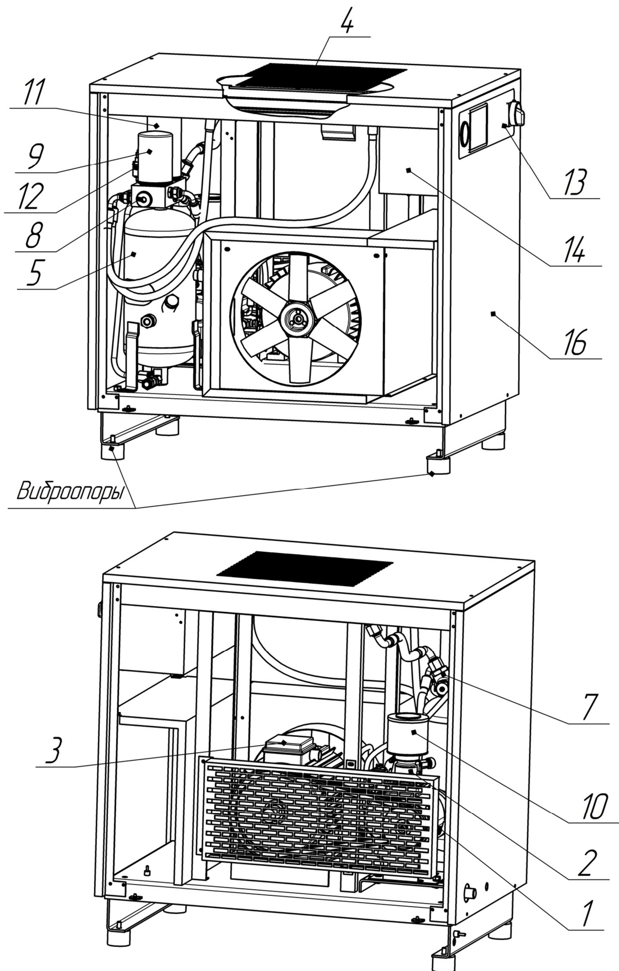
Рисунок 1 – Общий вид компрессорной установки ВК15Е-...
